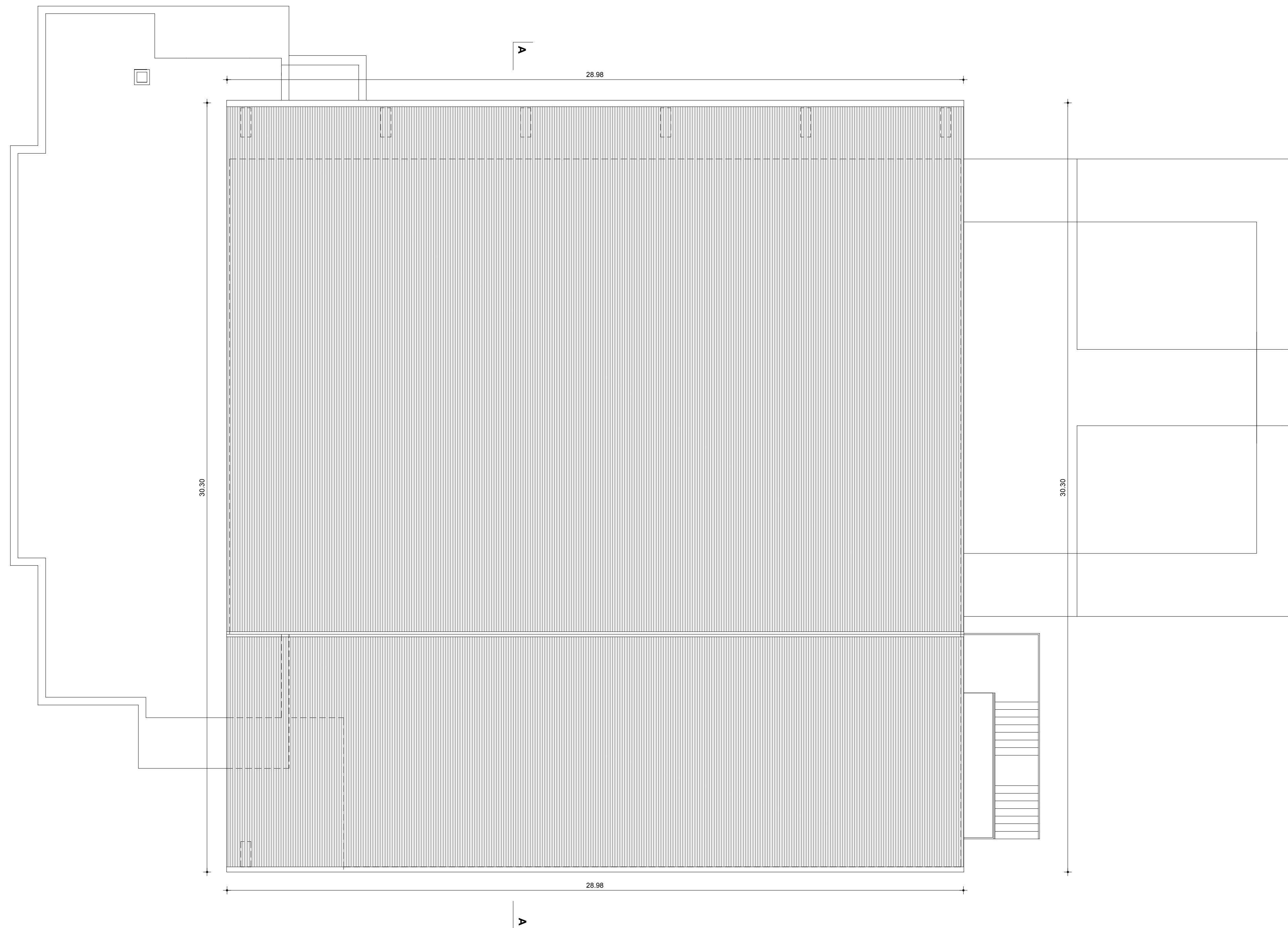
PIANTA COPERTURA
