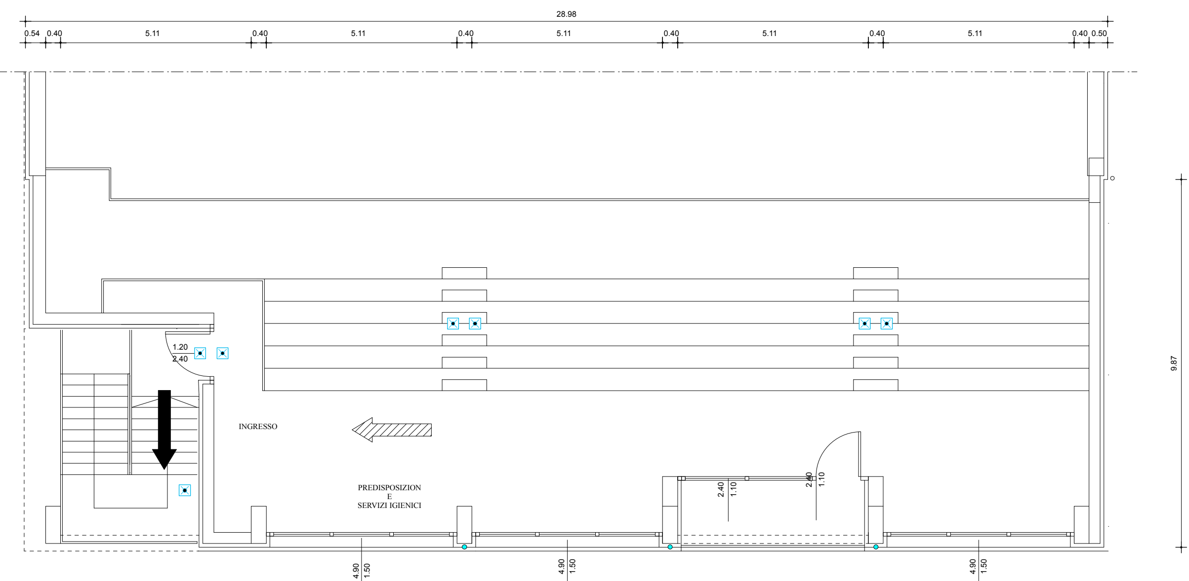
PIANTA QUOTA + 5.72 m scala 1:100
